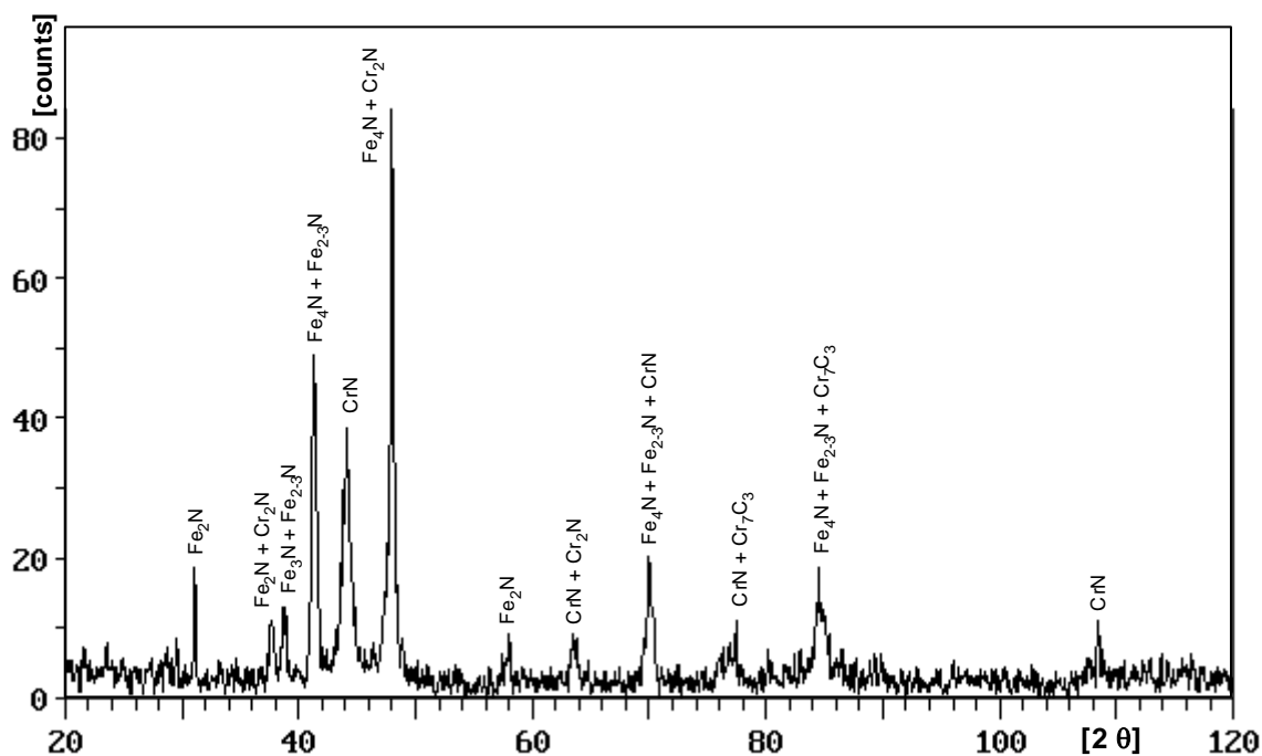
Figura 2 – Espectro de difração de Raios-X realizado na camada de compostos da amostra nitretada a 560°C.
