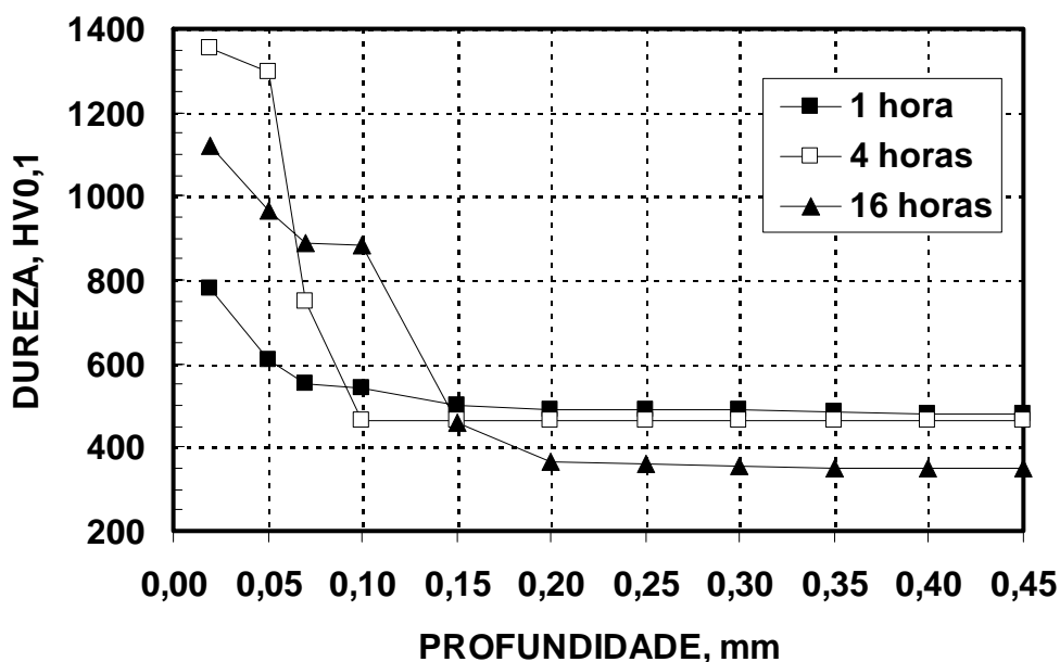
Figura. 4 – Perfis de microdureza determinados em cada condição de nitretação.
