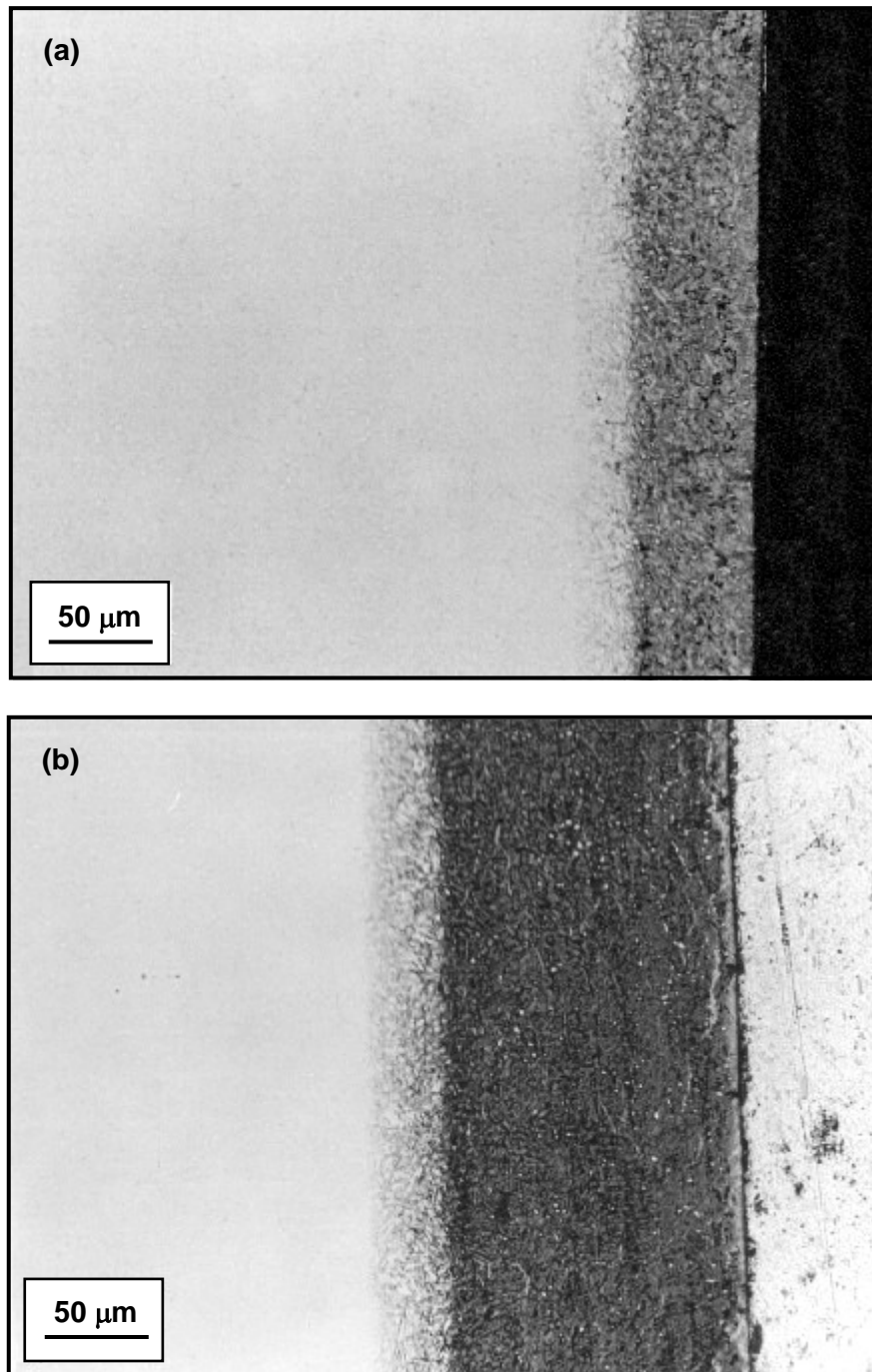
Figura. 1 – Microestruturas da superfície nitretada do aço AISI 420. Nitretação a 480°C (a) and 560°C (b). Nital 4%.
