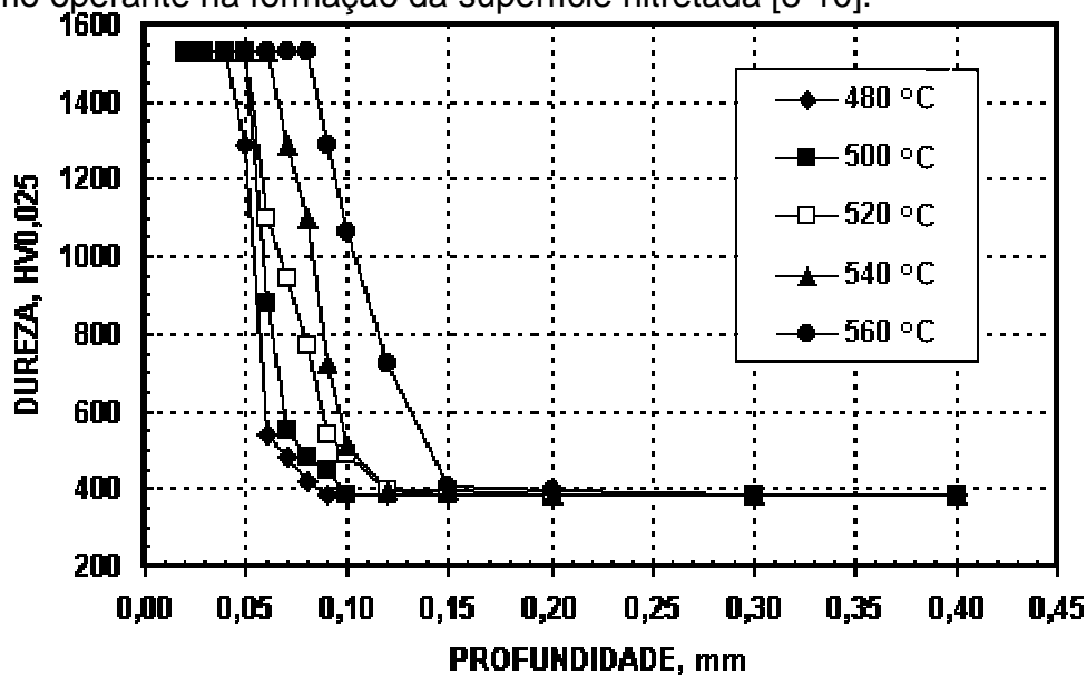
Figura 5 – Perfis de microdureza determinados para a série isotérmica.
