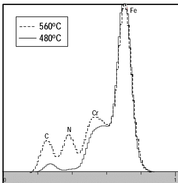
Figura 3 – Espectros de EDS em amostras nitretadas a 480 e 560°C, obtidos
